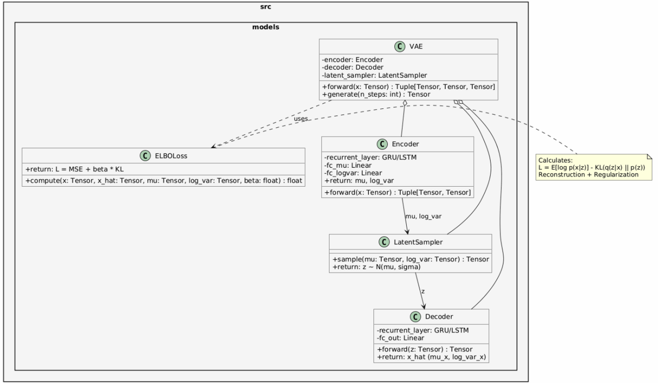
Рисунок 5 — Диаграмма классов модуля нейросетевых моделей
