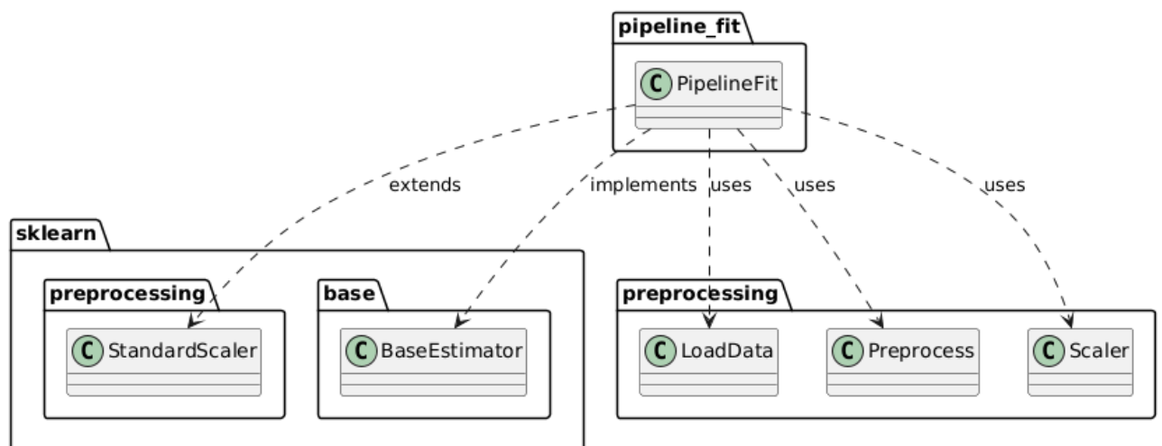
Рисунок 13 — Диаграмма классов модуля пайплайна
