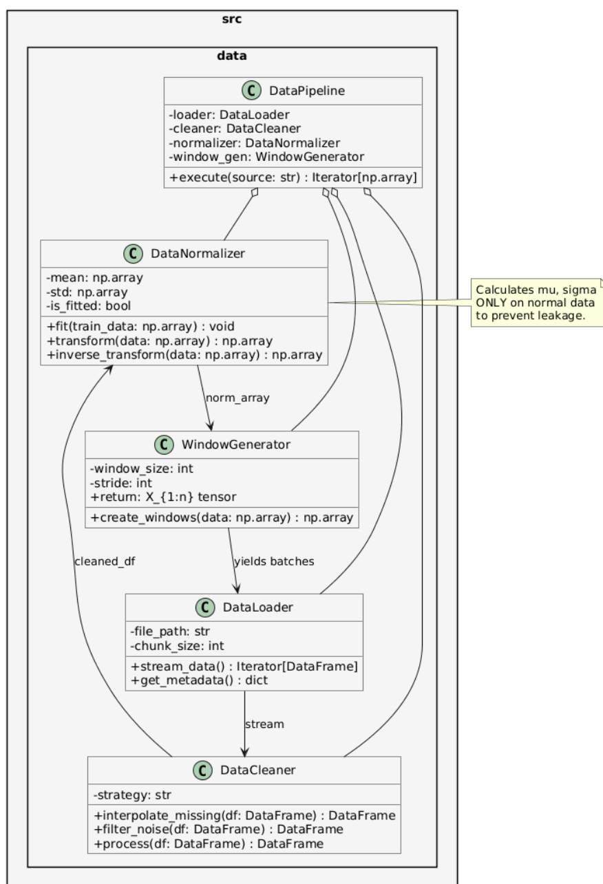
Рисунок 4 — Диаграмма классов модуля чтения и обработки данных
