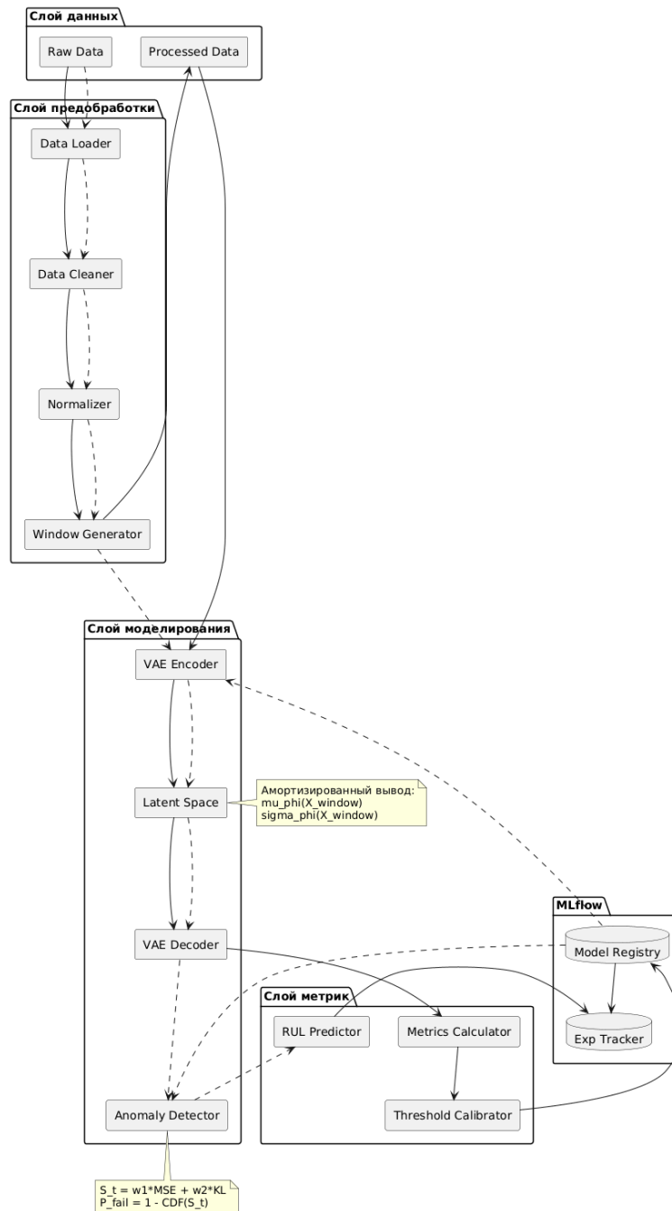
Рисунок 2 — Архитектура системы обучения и прогнозирования
