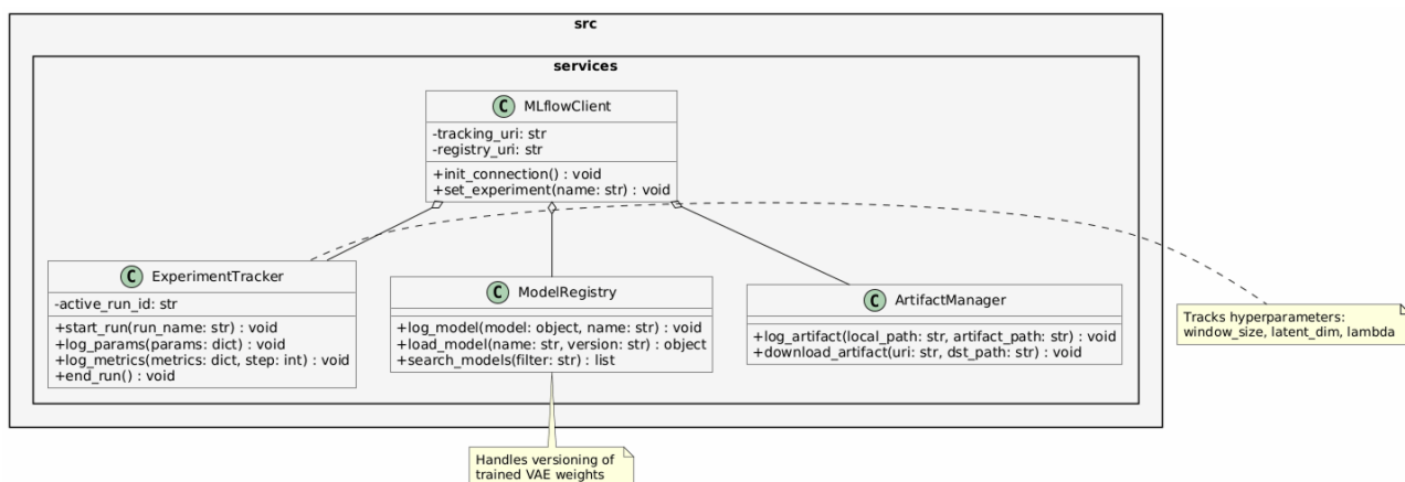
Рисунок 8 — Диаграмма классов модуля управления экспериментами
