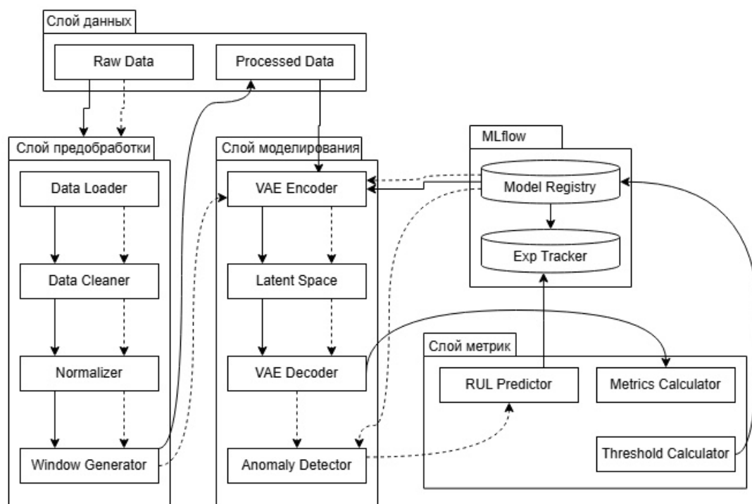
Рисунок 8 — Архитектура системы обучения и прогнозирования
