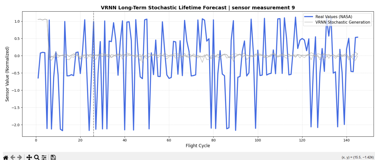
Рисунок 5 — Результат многошагового прогнозирования с использованием модели VRNN-VAE
