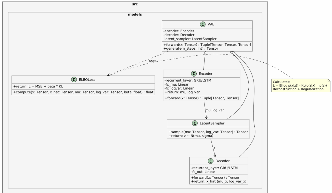
Рисунок 12 — Диаграмма классов модуля нейросетевых моделей
