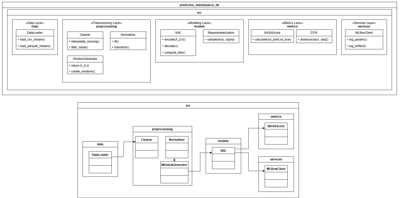
Рисунок 9 — Структура пакетов Python-библиотеки
