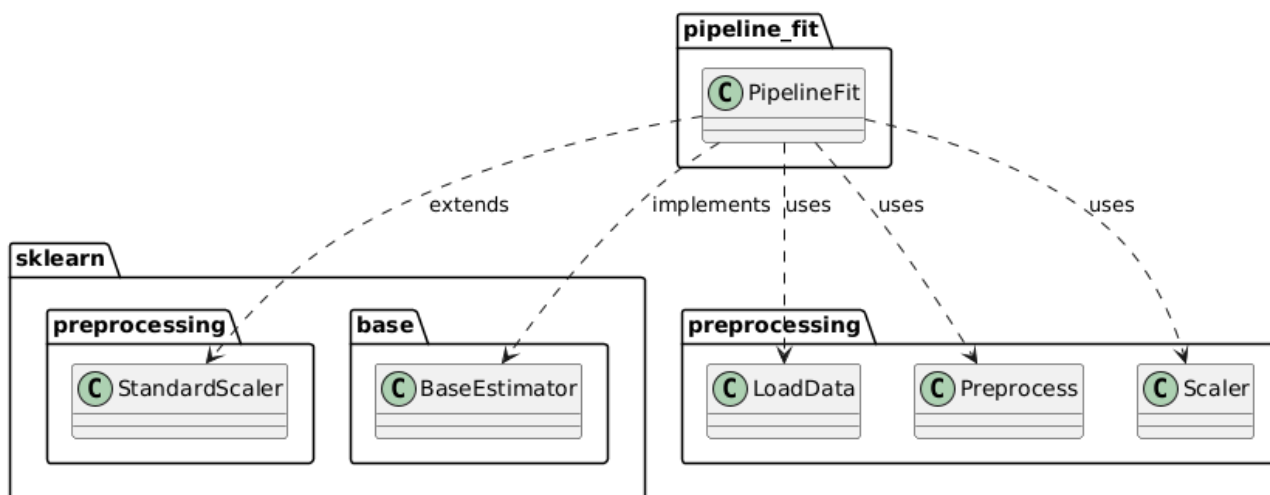
Рисунок 13 — Диаграмма классов модуля пайплайна
