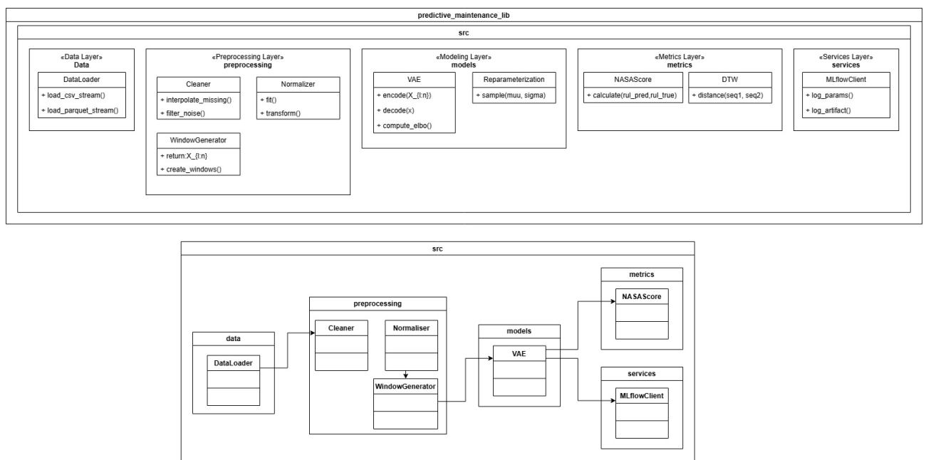
Рисунок 11 — Структура пакетов Python-библиотеки
