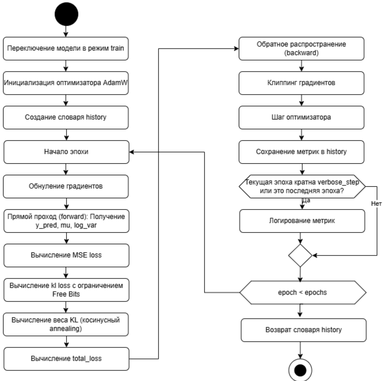
Рисунок 20 — Алгоритм работы метода fit()
