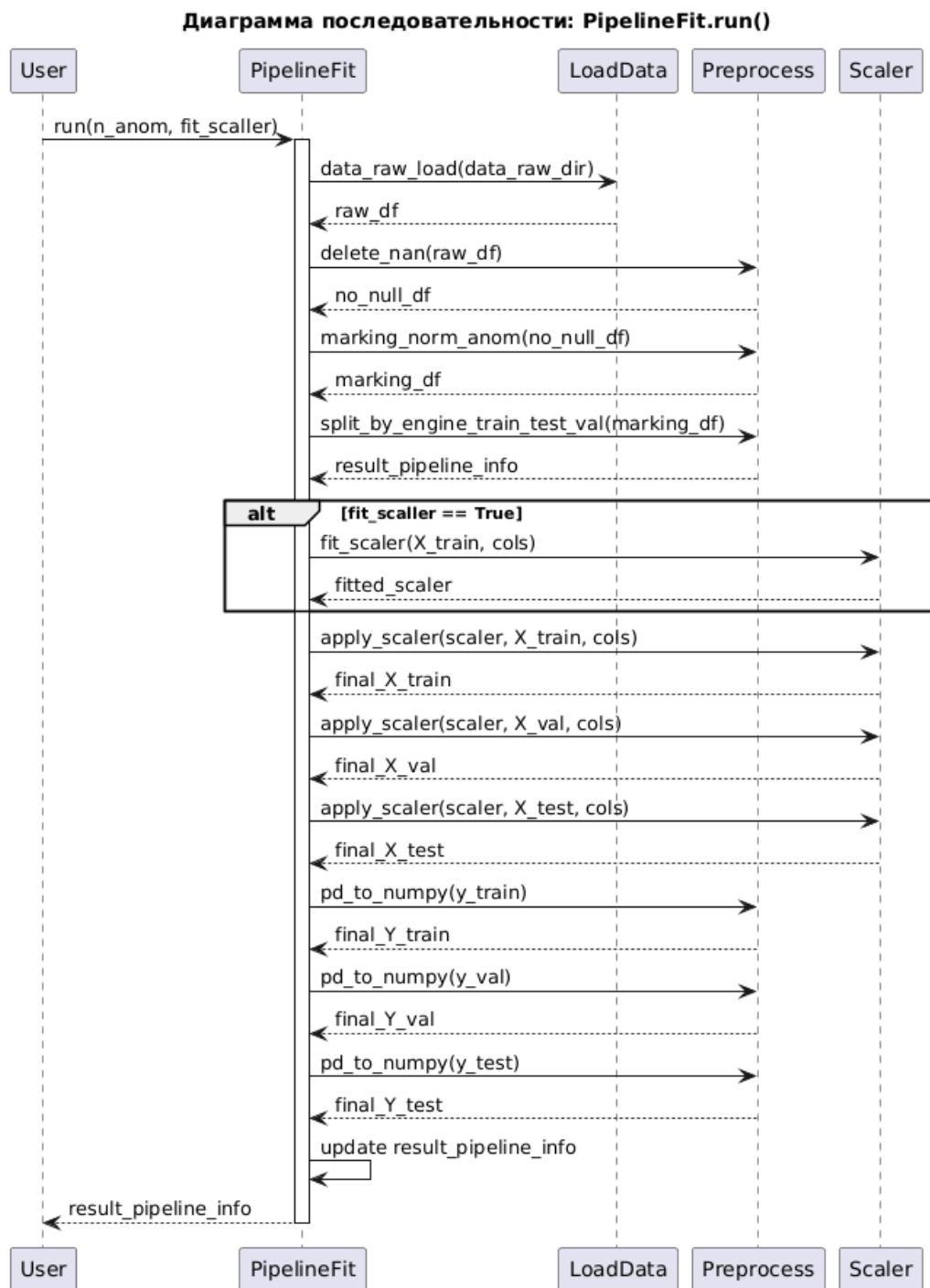
Рисунок 26 — Диаграмма последовательности взаимодействия компонентов системы
