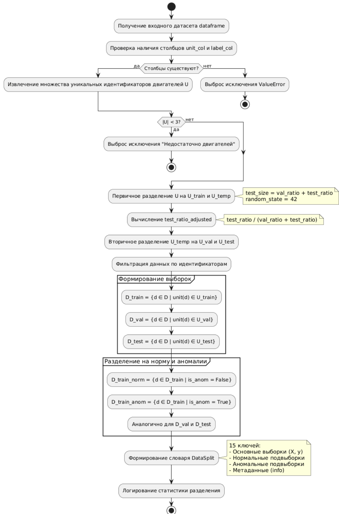
Рисунок 14 — Диаграмма алгоритма разделения исходных данных метода split_by_engine_train_test_val()
