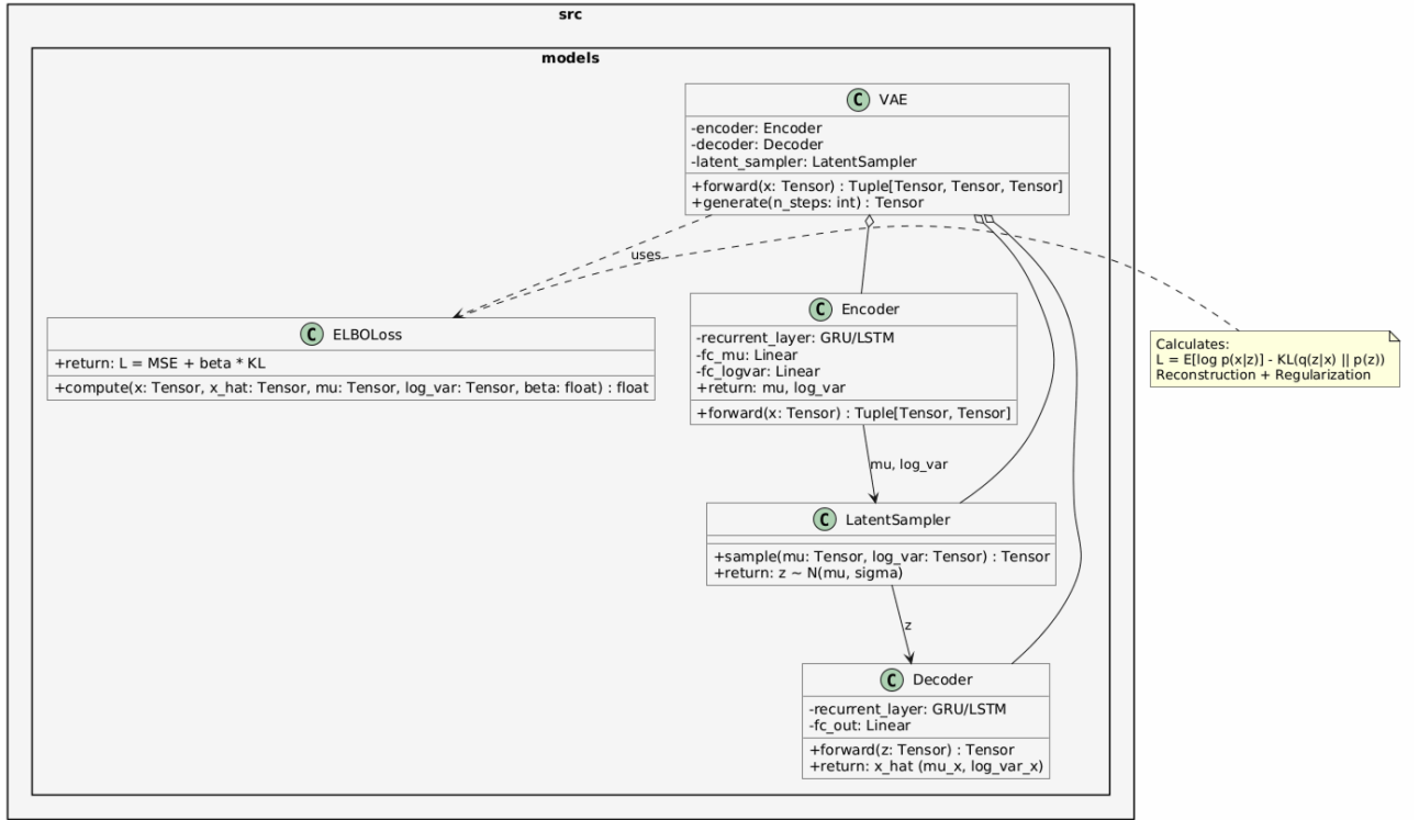
Рисунок 6 — Диаграмма классов модуля нейросетевых моделей
