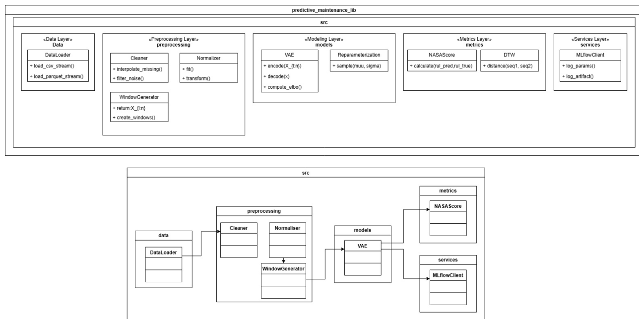
Рисунок 3 — Структура пакетов Python-библиотеки
