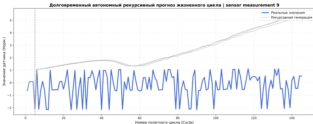
Рисунок 7 — Результат многошагового прогнозирования с использованием модели SSM-VAE
