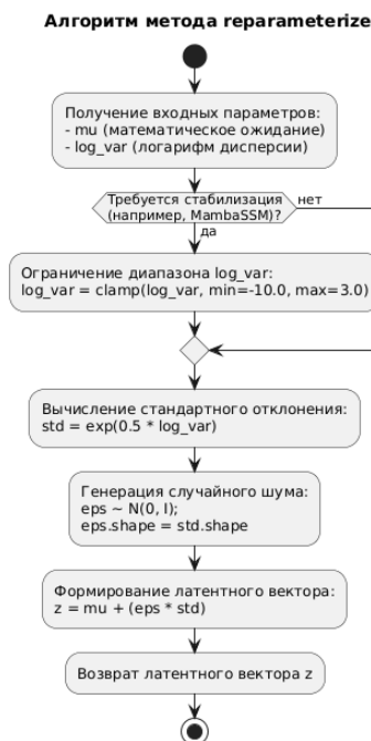
Рисунок 18 — Алгоритм работы метода reparameterize()
