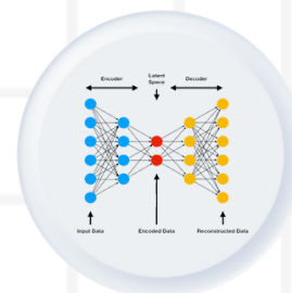
Autoencoders
