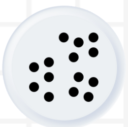
t-SNE
