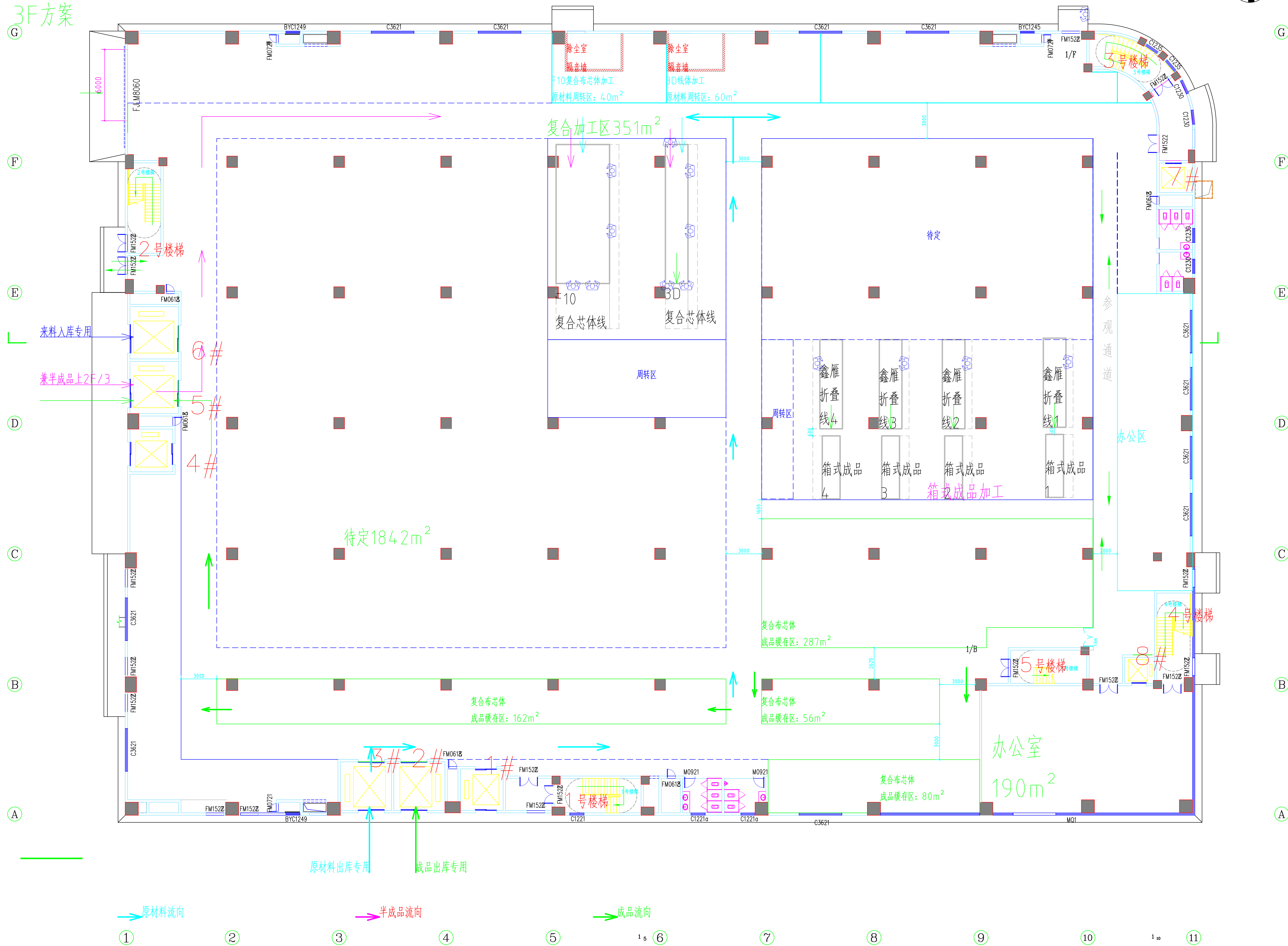
2#厂房3F规划俯视图:
