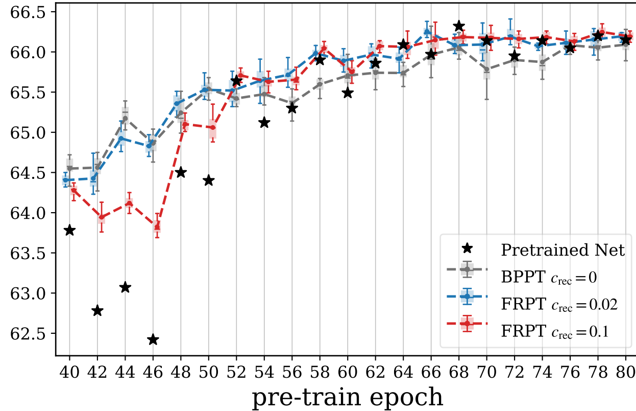
epoch10 testacc (%)
