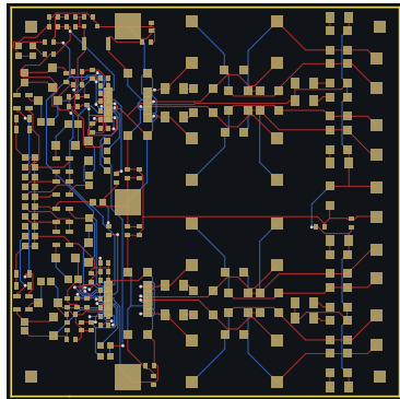
FR 2.5.0-RC12 · 7 DRC errors
