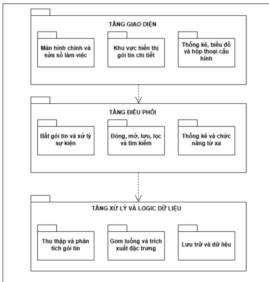
Hình 4.1: Biểu đồ gói UML của hệ thống
