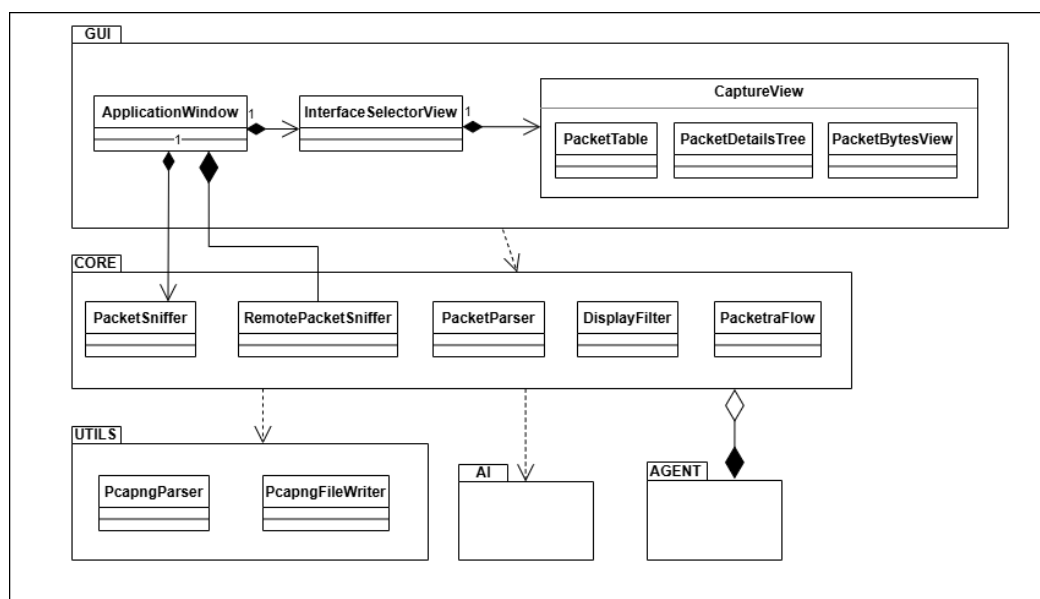
Hình 4.2: Biểu đồ thiết kế chi tiết gói của hệ thống
