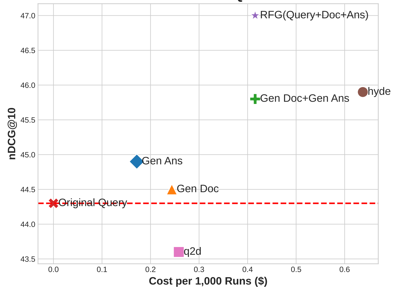
Dataset: ARGUANA
