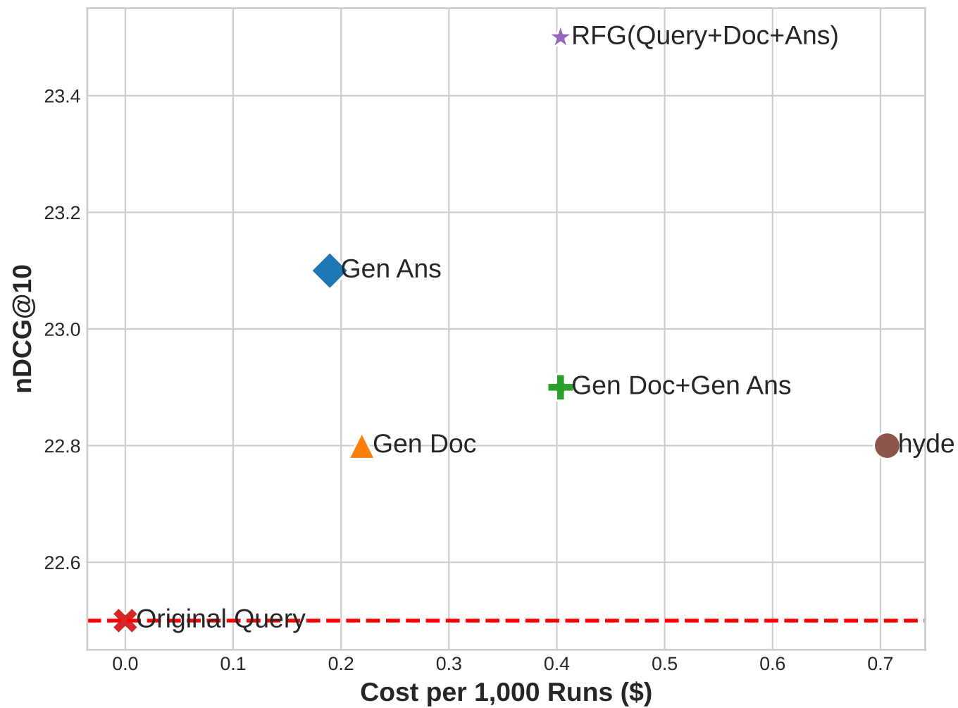
Dataset: SCIDOCS
