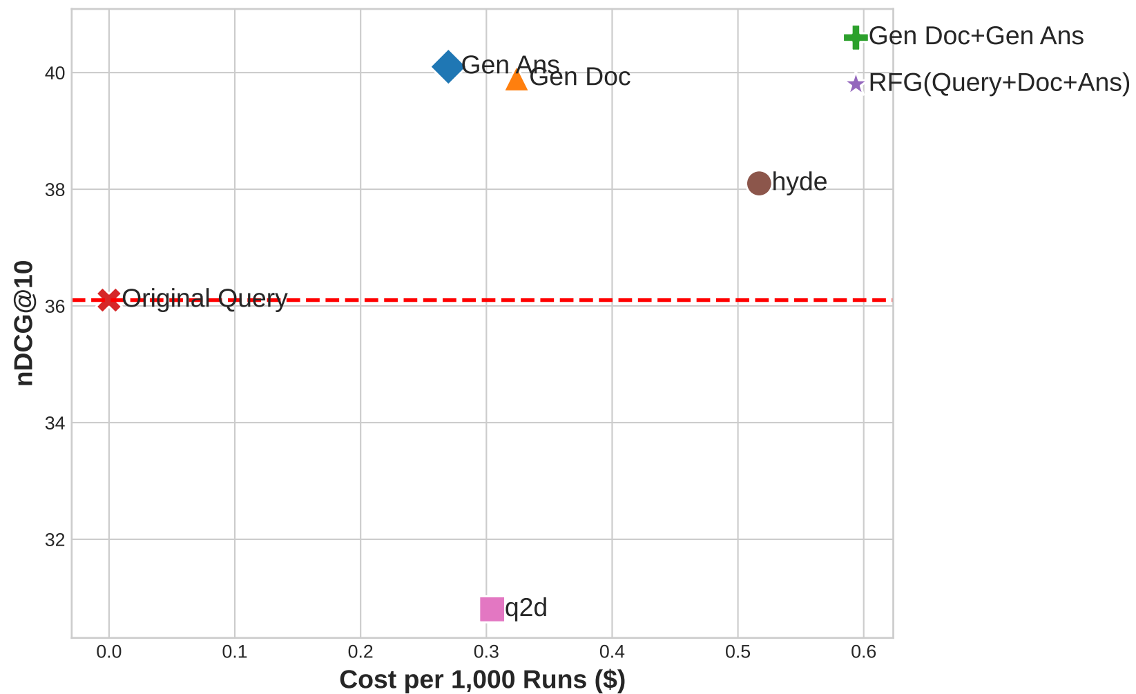
Dataset: SCIDOCS
