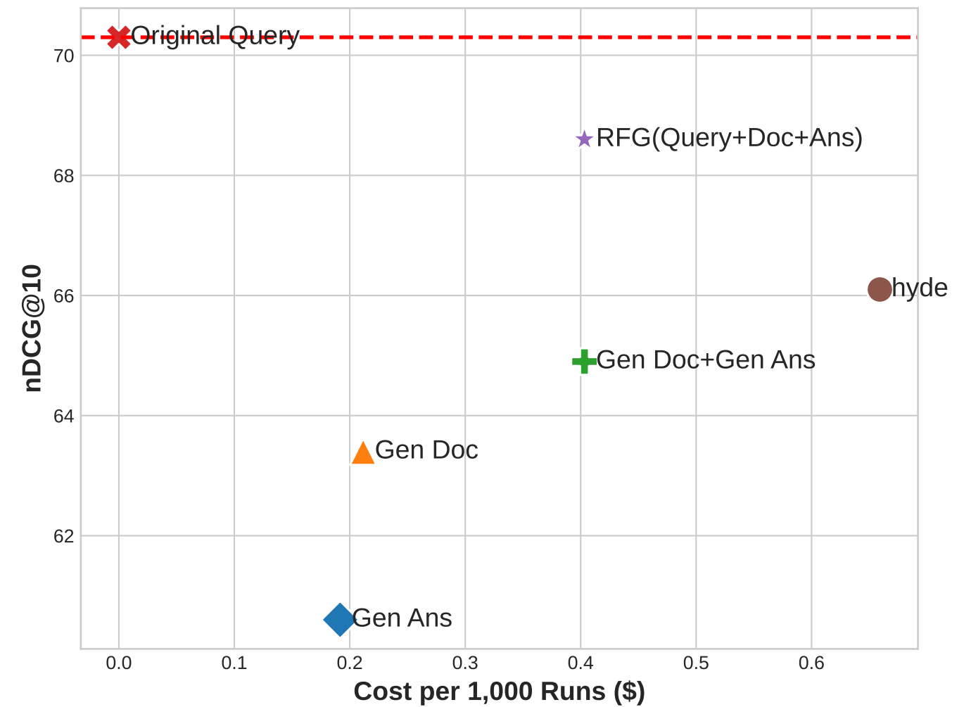
Dataset: ARGUANA
