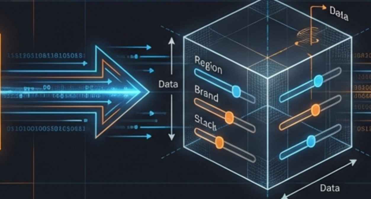
Parameterised Templates
