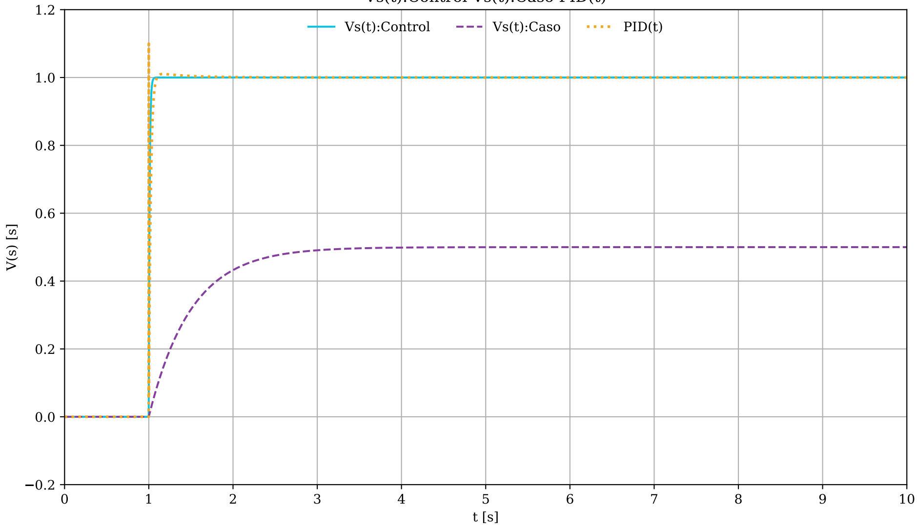
Vs(t):Control Vs(t):Caso PID(t)
