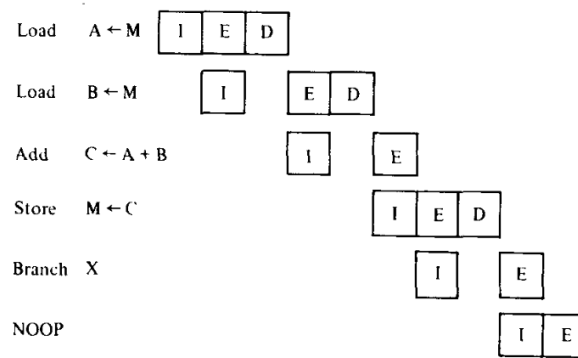
Figura 17 – Demonstração da pipeline do RISC I.(STALLINGS, 1988)
