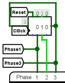
Figura 29 – Contador em Anel, implementado com um Registrador de Deslocamento de 3 bits
