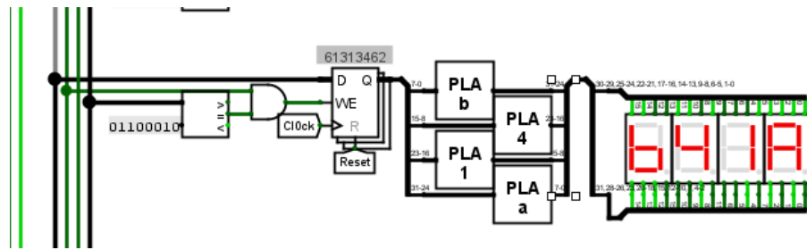
Figura 51 – Decodificador de display de sete segmentos no Logisim Evolution.
