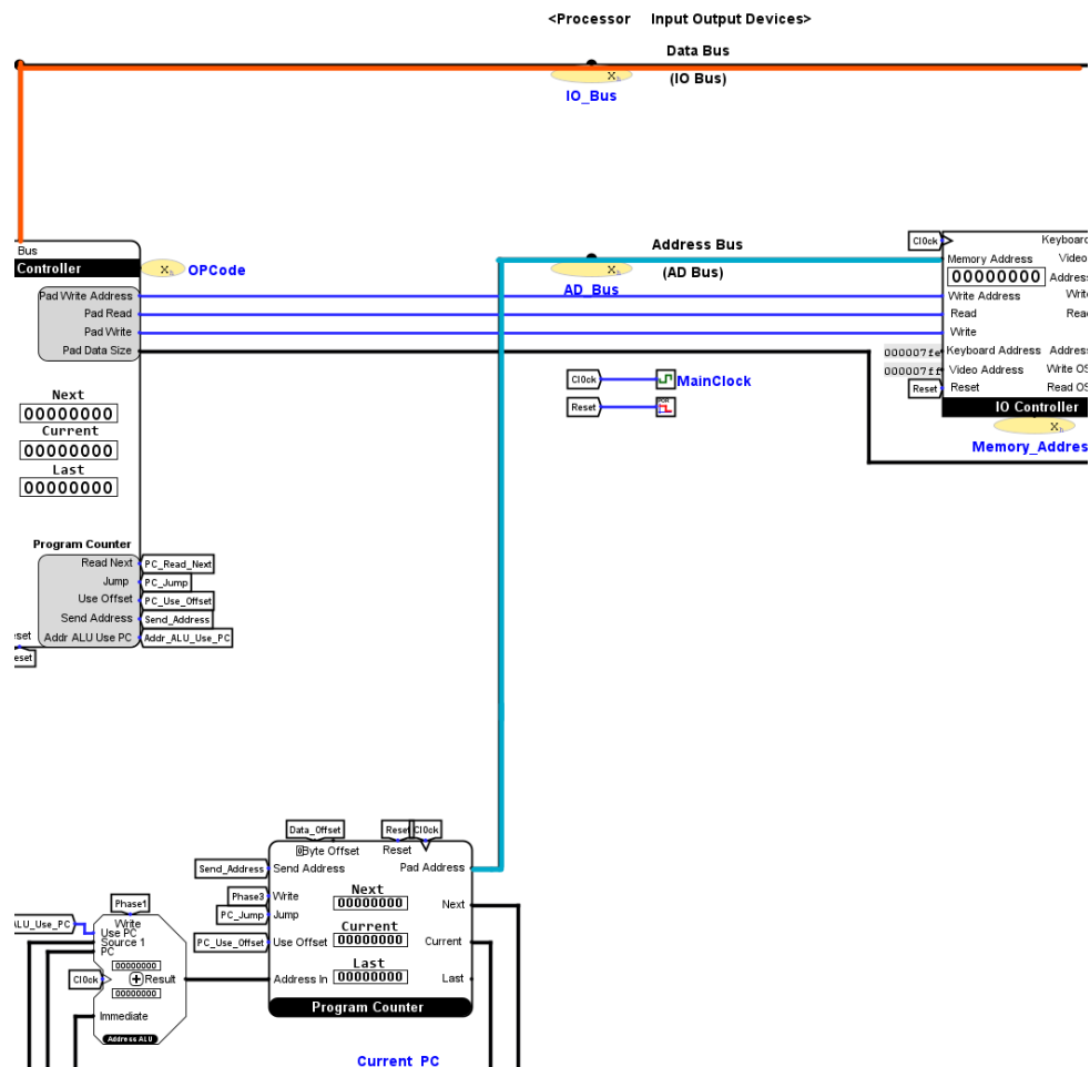
Figura 26 – Separação dos barramentos de dados e endereços
