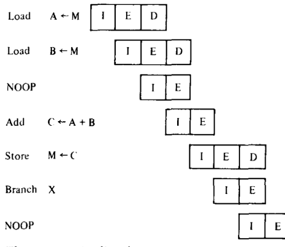
Figura 18 – Demonstração da pipeline do RISC II.(STALLINGS, 1988)
