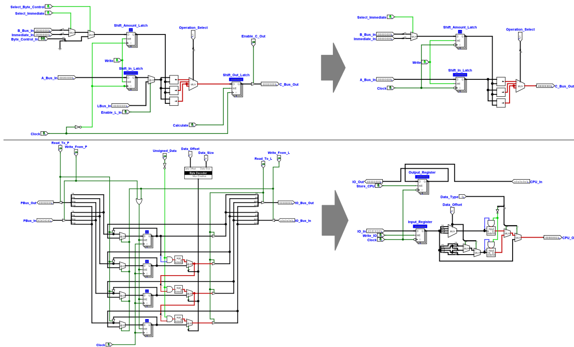
Figura 24 – Comparação entre o Deslocador (acima) e o DataIO (abaixo) antes e depois
