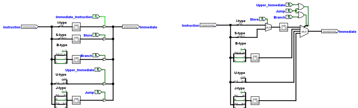
Figura 20 – Comparação entre o Decodificador de Imediato com buffers tri-state (esquerda) e multiplexadores (direita)
