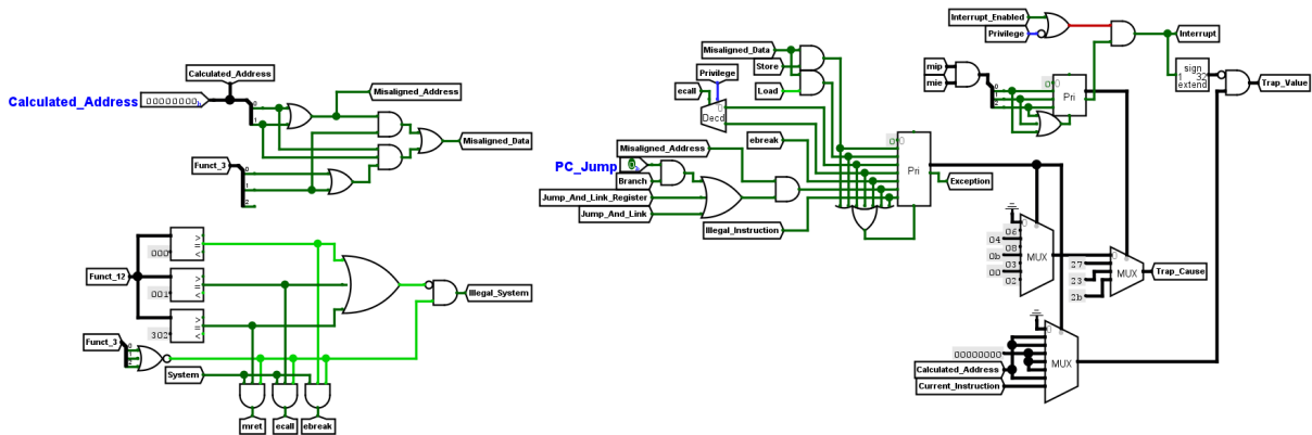
Figura 40 – Circuitos de tratamento de traps .
