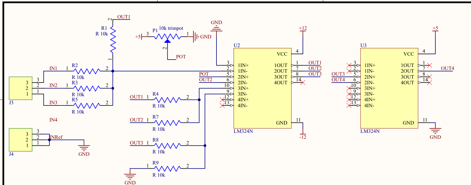
Amplificadores
