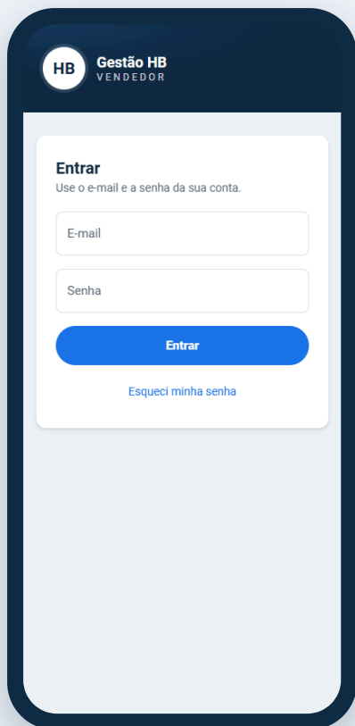
Login
