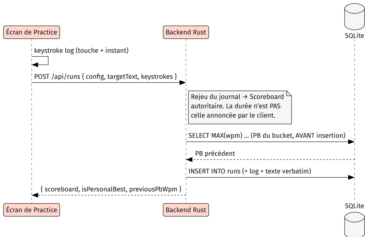
Figure 41. – La soumission d'un Run solo. L'ordre compte : le PB précédent est lu avant l'insertion, sinon le Run qu'on vient d'écrire serait son propre record à battre et aucun record ne serait jamais annoncé.
