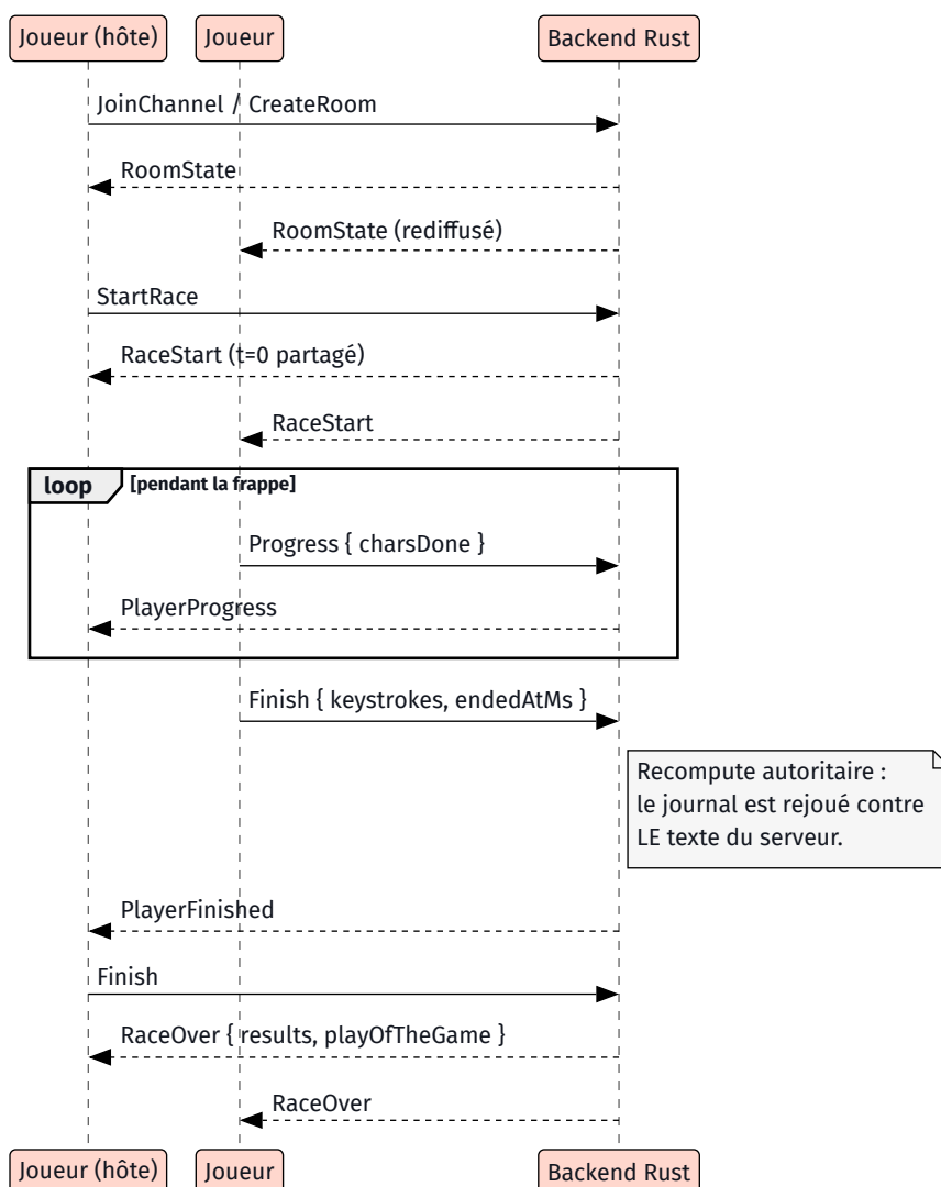
Figure 38. – Une Race normale. Le RaceOver ne part qu'une fois le dernier journal attendu arrivé — c'est pourquoi un abandon débloquent les autres au lieu de les faire patienter jusqu'au watchdog. Les deux Finish sont recomputés séparément ; le classement, lui, se décide en une seule fois.
