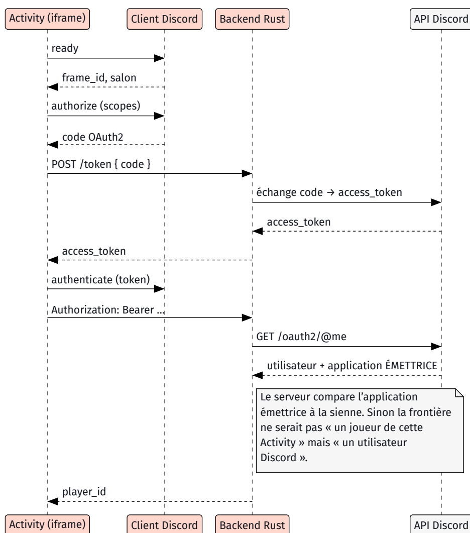
Figure 18. – Le handshake d'identité. Le secret client ne quitte jamais le serveur : c'est lui, et non l'iframe, qui échange le code contre un jeton. La dernière vérification est celle qui compte — un jeton d'accès Discord est valable sur l'endpoint d'identité quelle que soit l'application qui l'a obtenu (issue 150).
