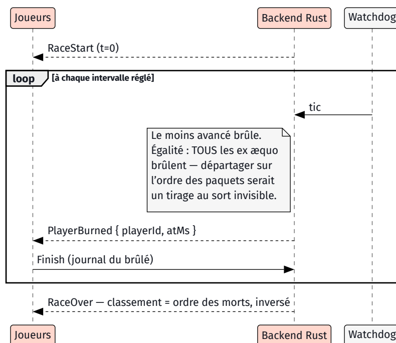
Figure 39. – Floor is lava. Le métronome part au signal de départ partagé et non à la création de la course : sinon le premier battement tomberait pendant le décompte, où personne n’a encore tapé — tout le monde est dernier, tout le monde brûle (issue 159). La course s’arrête à un vivant ; à zéro vivant, une égalité finale a emporté les deux derniers et il n’y a pas de vainqueur.
