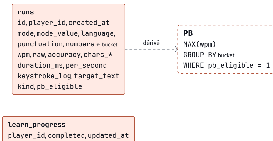
Figure 40. – Le schéma. Le PB est encadré en pointillés parce qu'il n' existe pas : c'est une requête, pas une ligne. Un record ne peut donc jamais désigner un Run qui n'est plus là, ni survivre à une règle d'éligibilité qui change.
