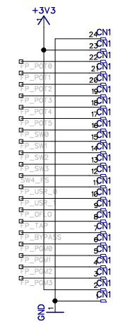
FH12-24S-0.5SH(55)
