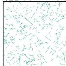
LCO 1 m · 타원율 중앙 0.046 · 장축-방사각 42°
