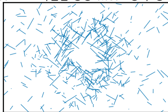
CDK 508 mm · 타원율 중앙 0.039 · 장축-방사각 42°
