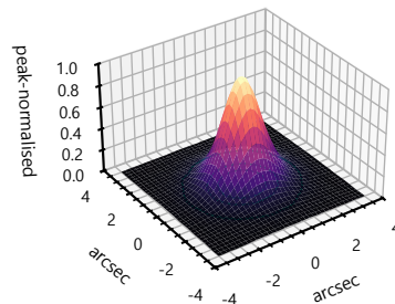
LCO 1 m (RC 계열) — NGC 5985, rp
