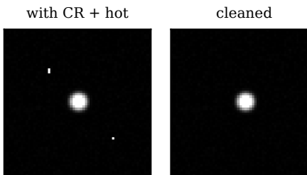
(d) Cosmic-ray + hot-pixel removal
