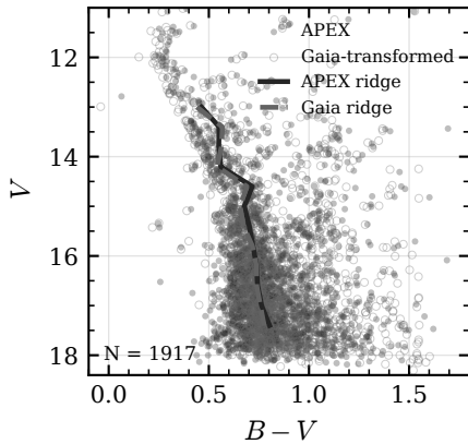
(c) CMD ridge RMS 19 mmag
