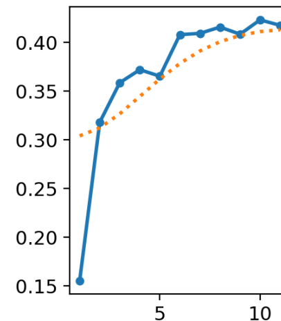
metrics/mAP50-95(B)
