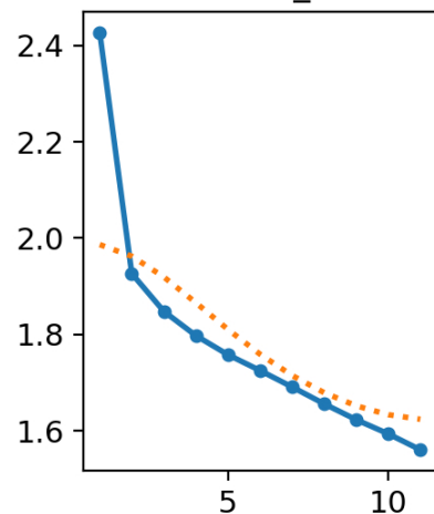
val/box_loss
