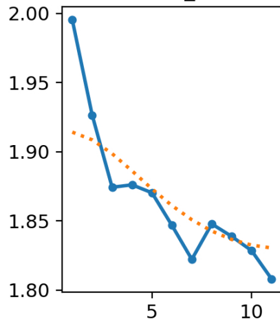
val/box_loss
