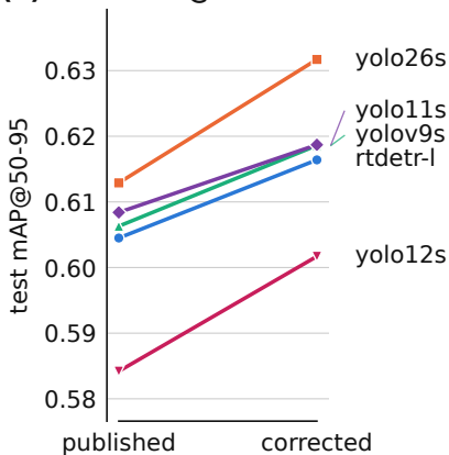
(b) test mAP@50-95
