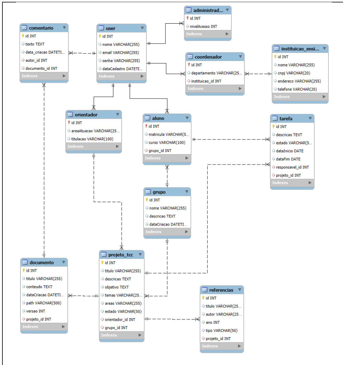
Figura 6 – Exemplo: Modelo Relacional gerado por engenharia reversa (MySQL Workbench).
