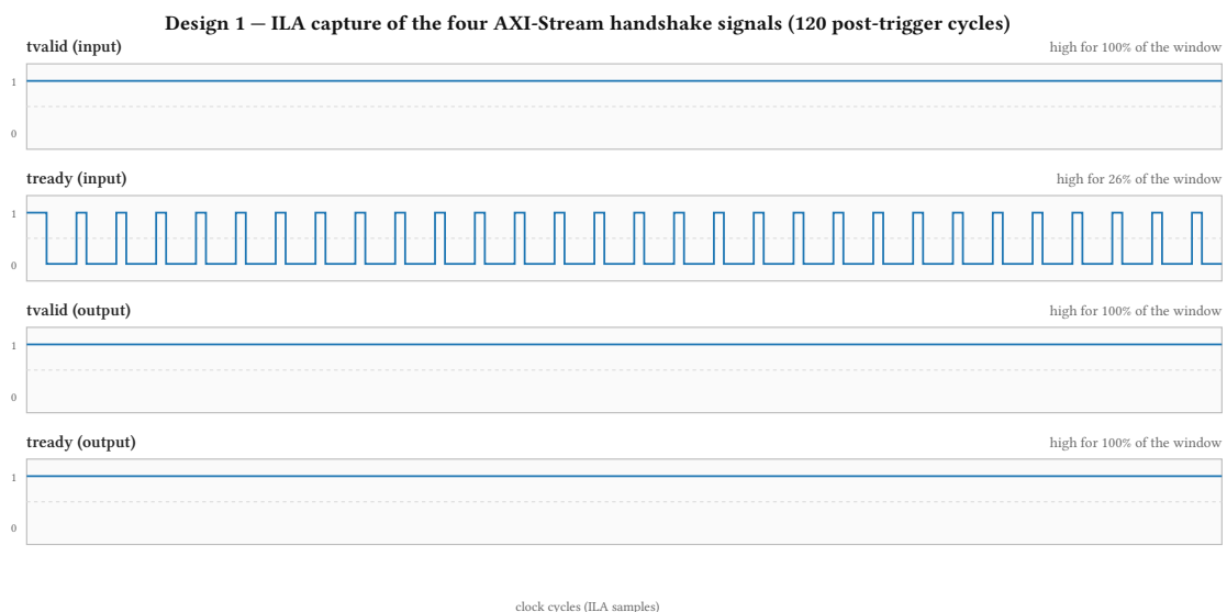
Figure 3: Capture ILA des quatre signaux de handshake AXI-Stream du Design 1, à 250 MHz, sur 120 cycles post-trigger. Le tready de l'entrée est le seul signal qui pulse ; les trois autres restent collés à 1 sur toute la fenêtre.
