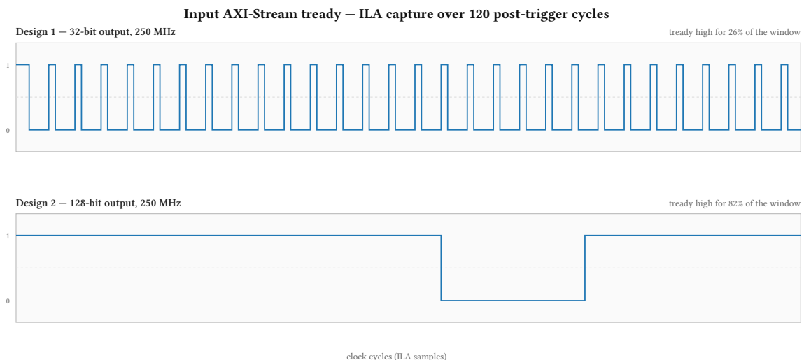
Figure 4: Capture ILA du signal tready de l'AXI-Stream d'entrée sur le Design 1 (haut) et le Design 2 (bas), à 250 MHz. Sur le Design 1, le signal pulse périodiquement (un cycle haut sur quatre) ; sur le Design 2, il reste à 1 la quasi-totalité du temps. La fenêtre affichée couvre 120 cycles post-trigger ; les ratios cités dans le texte (20.9 % / 88.7 %) sont calculés sur la fenêtre complète de 512 échantillons.
