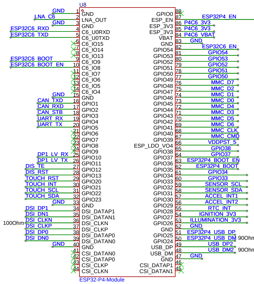
ESP32-P4-Module (Waveshare)
