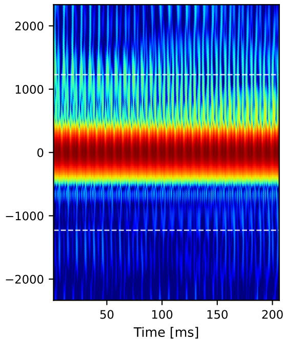
Sionna PathSolver 7.7 dB p-p · level -60 dB vs strongest
