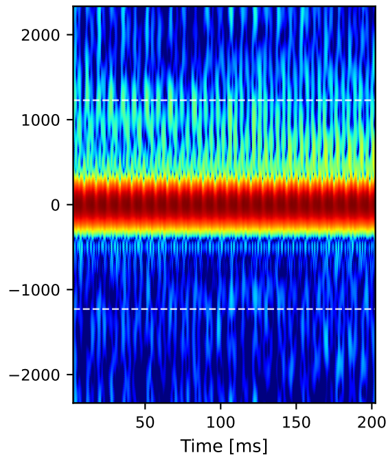
Sionna PathSolver 6.8 dB p-p · level -60 dB vs strongest
