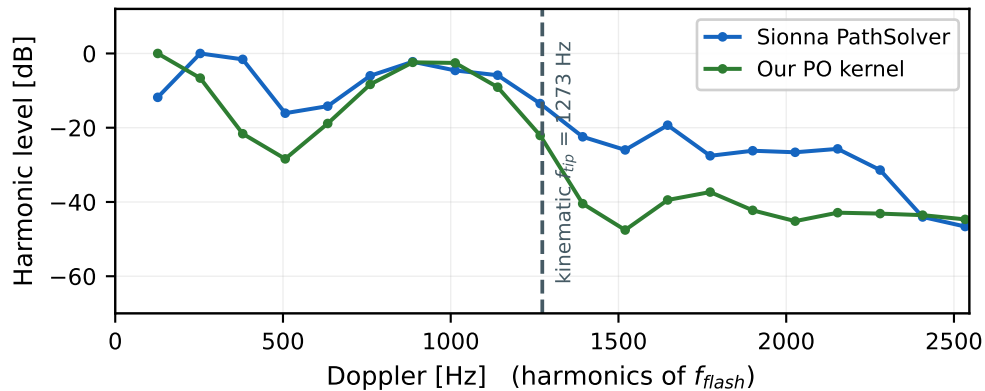
DJI Matrice 4E — harmonic comb, 3800 rpm
