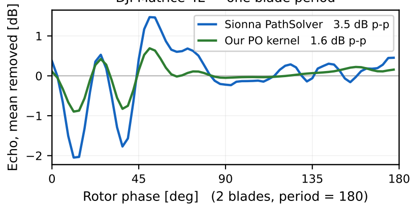
DJI Matrice 4E — one blade period
