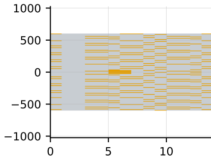
LTE Rel-9 G3 - PRS
