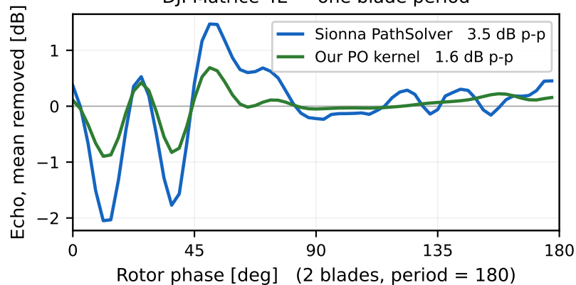
DJI Matrice 4E — one blade period
