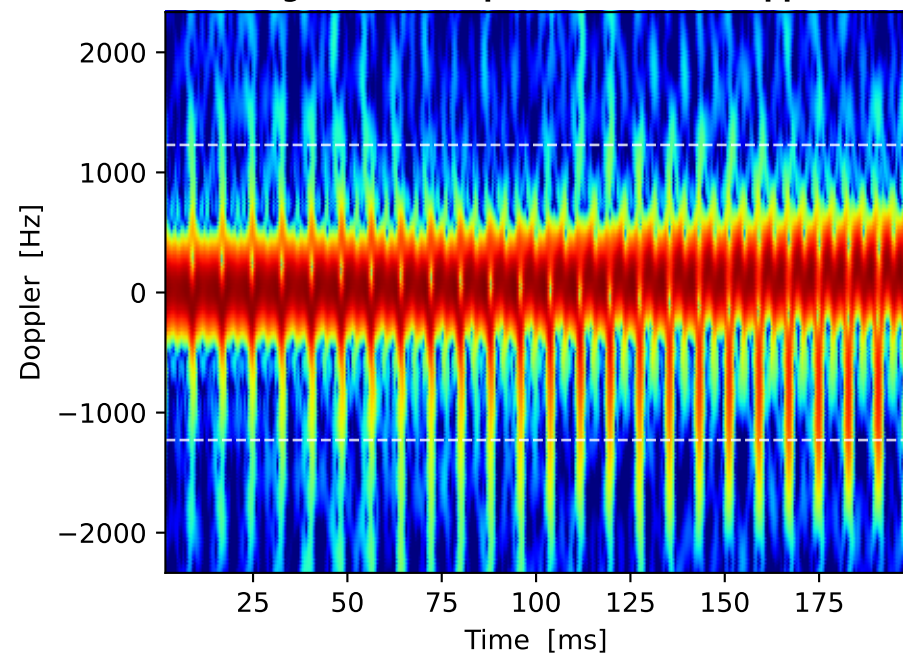
(d) Ledger STFT (no passive chain) — upper bound
