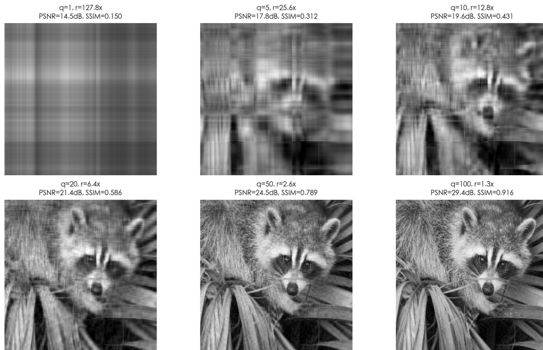
SVD rank-q 影像重建
