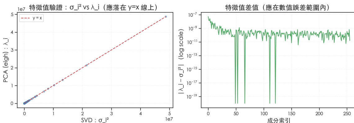
PCA 等價性驗證 (a) : 特徵值比較
