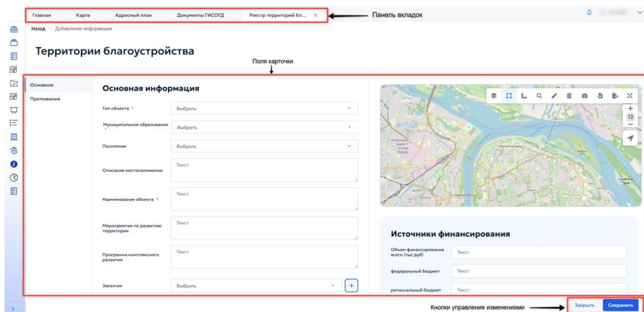
Рисунок 11 — Основные элементы карточки.
