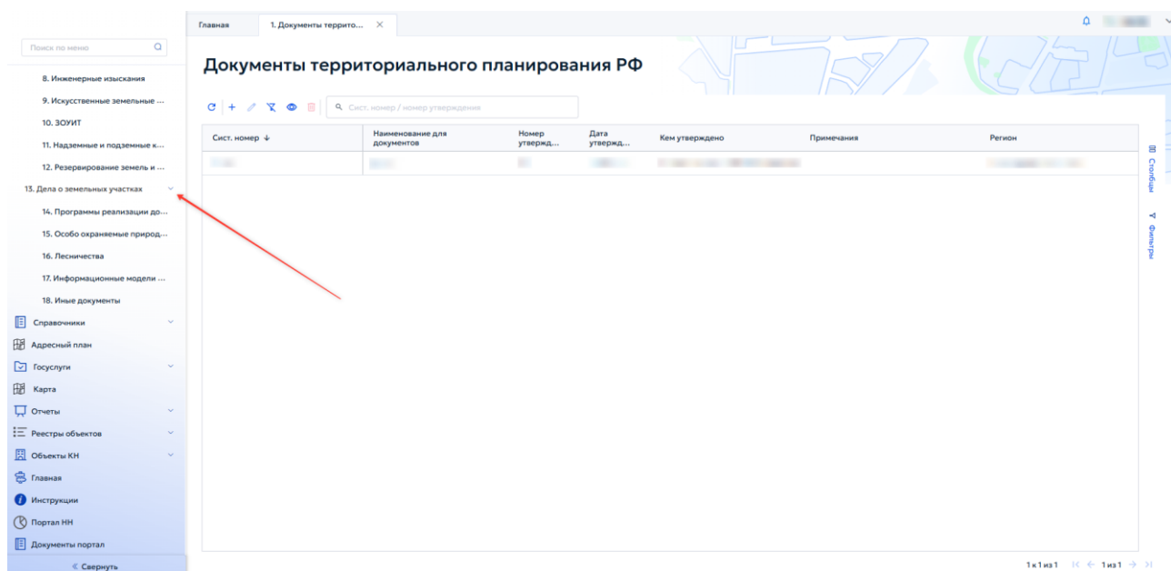
Рисунок 5 — Работа с группировочным пунктом меню.
