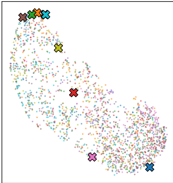
single-latent CS-WAE
