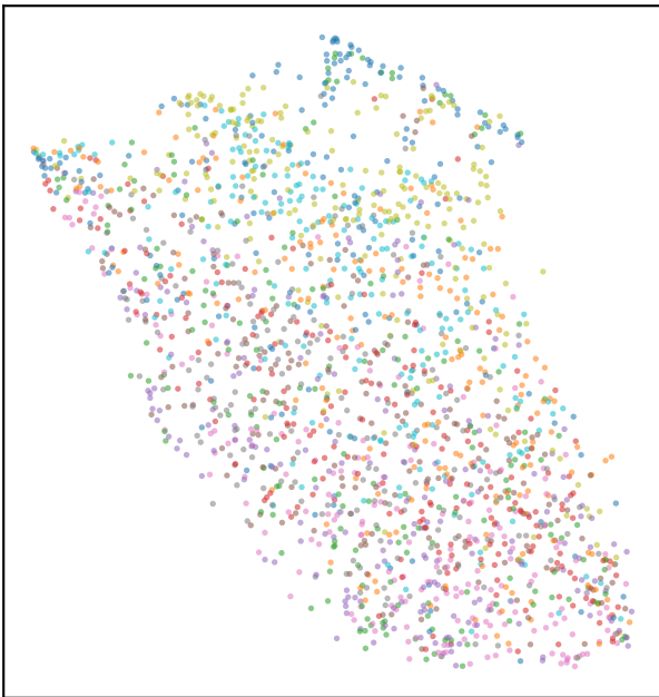
AE latent
