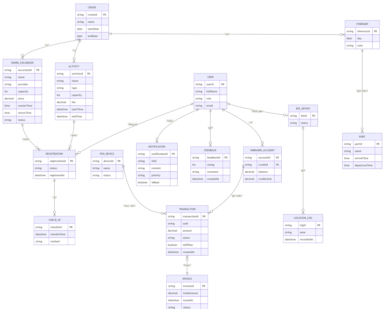
Hình 3.10: Sơ đồ ERD mức khái niệm
