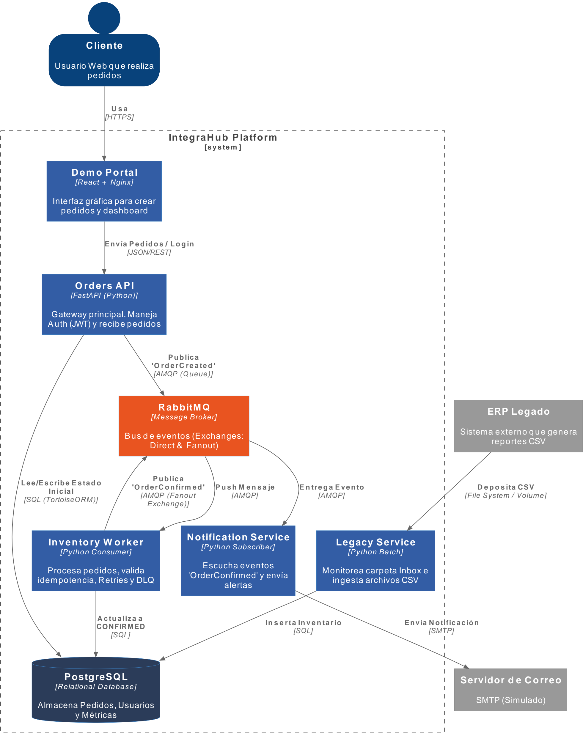
Diagrama de Contenedores C4 - IntegraHub Platform
