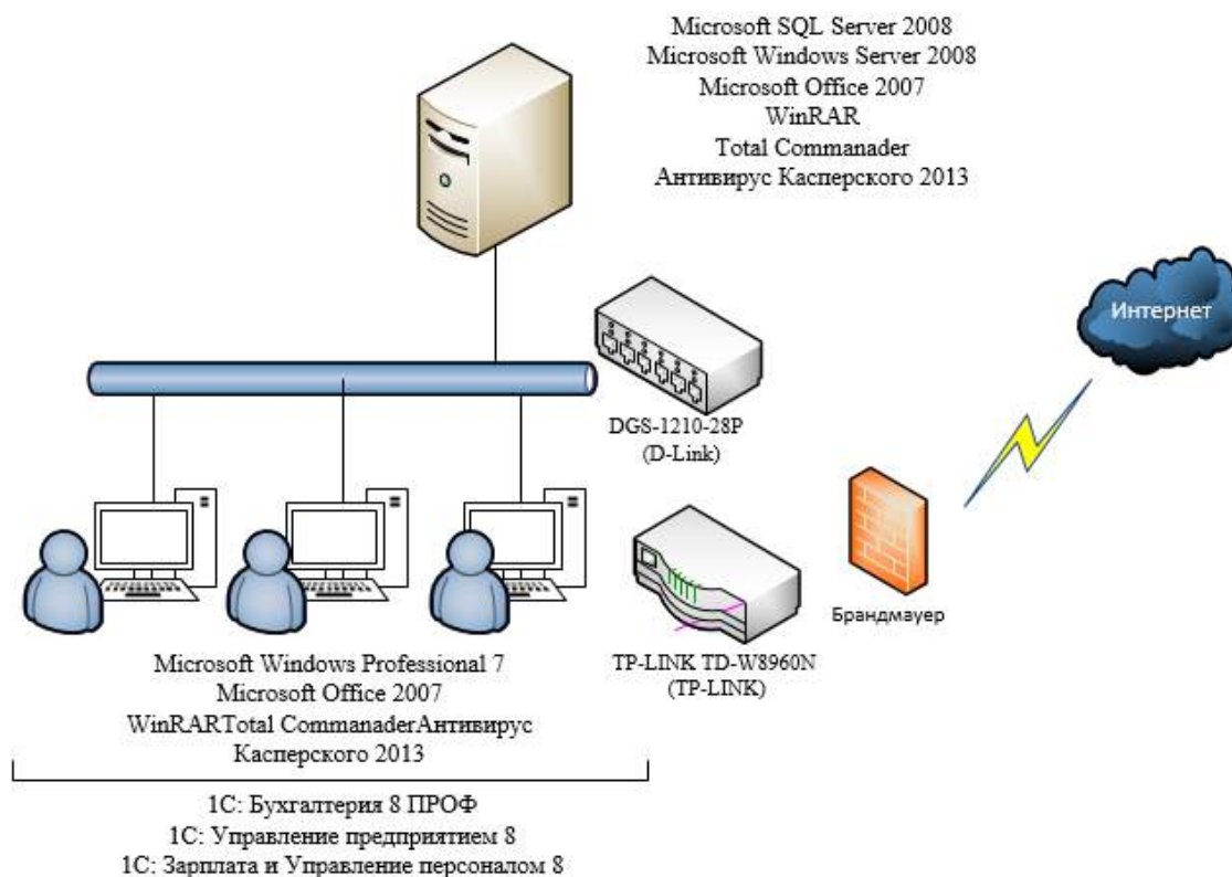
Рис. 1.8. Схема ЛВС ООО «СиВер»
