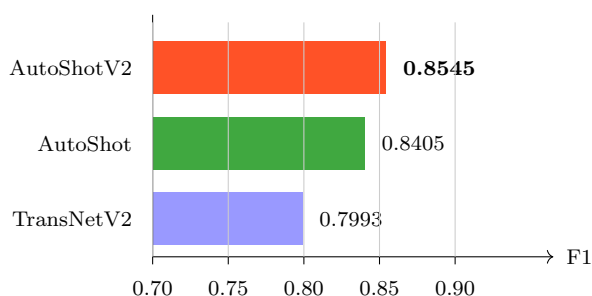
Hình 4.3: So sánh F1 giữa các mô hình trên tập SHOT (200 video kiểm tra). AutoShotV2 đạt F1 = 0.8545 , cải thiện +1.4\% so với AutoShot gốc và +5.5\% so với TransNetV2 mô hình cơ sở.
