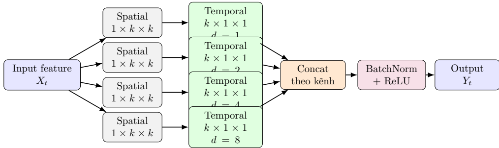
Hình 3.4: Cấu trúc chi tiết của khối DDCNN trong TransNetV2: 4 nhánh tích chập thời gian 1D với độ giãn nở d \in \{1, 2, 4, 8\} song song nhau, đầu ra được nối ghép theo chiều kênh. Mỗi nhánh trước tiên qua tích chập không gian 2D ( 1 \times k \times k ) rồi mới qua tích chập thời gian 1D giãn nở ( k \times 1 \times 1 ).
