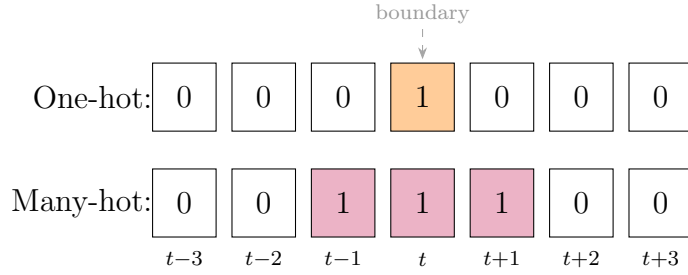
Hình 3.9: Minh họa nhãn one-hot và many-hot. Nhãn one-hot chỉ gán 1 tại đúng khung ranh giới t ; nhãn many-hot mở rộng thêm t \pm 1 , cung cấp tín hiệu gradient dày đặc hơn quanh vùng ranh giới.
