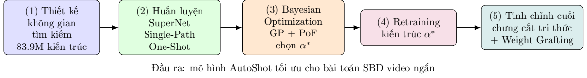
Hình 3.6: Sơ đồ 5 pha của quy trình NAS trong AutoShot: (1) Thiết kế không gian tìm kiếm với 83.9M kiến trúc; (2) Huấn luyện SuperNet theo chiến lược Single-Path One-Shot; (3) Tìm kiếm kiến trúc tối ưu bằng Bayesian Optimization (GP + PoF); (4) Huấn luyện lại kiến trúc \alpha^* ; (5) Tinh chỉnh bằng chưng cất tri thức và Weight Grafting.
