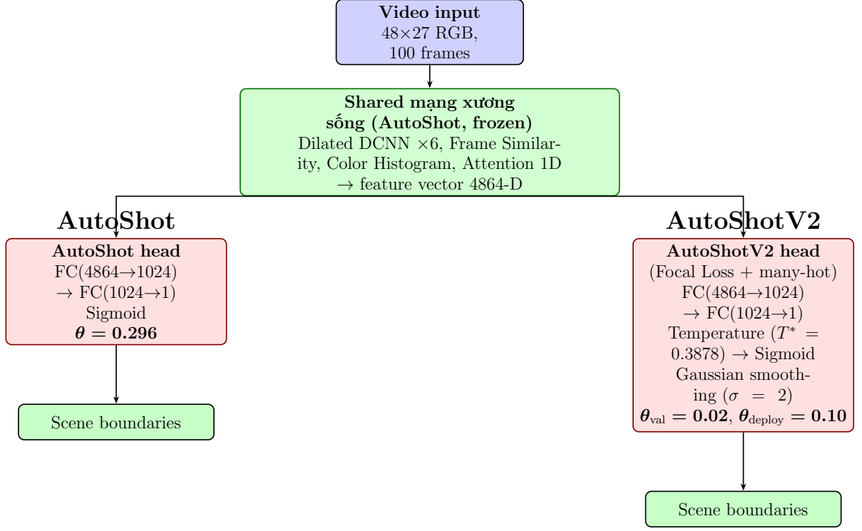
Hình 4.3: Sơ đồ khối so sánh AutoShot và AutoShotV2. mạng xương sống đã được NAS tối ưu (khung xanh) được đóng băng và chia sẻ cho cả hai mô hình; điểm khác biệt nằm hoàn toàn ở tầng phân loại và hậu xử lý (khung đỏ). So với AutoShot, AutoShotV2 huấn luyện lại tầng phân loại với Focal Loss + nhãn many-hot, thêm temperature scaling trên logit, Gaussian smoothing trên chuỗi xác suất, và sử dụng ngưỡng tối ưu trên validation sau hiệu chỉnh. Kiến trúc chi tiết từng thành phần xem Mục 3.5 của Chương 3.
