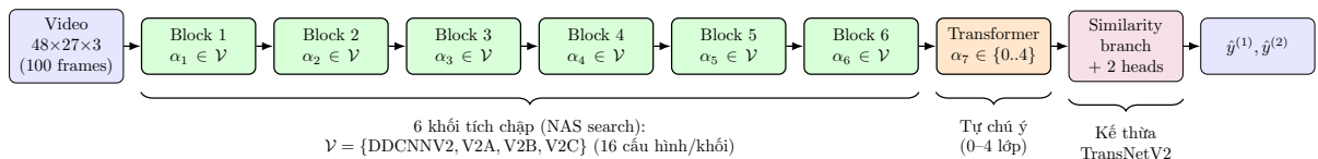
Hình 3.4: Sơ đồ tổng thể mô hình AutoShot gồm 7 vị trí kiến trúc cần tìm kiếm. Sáu vị trí đầu là các khối tích chập phân tách 3D chọn từ \mathcal{V} = \{\text{DDCNNV2, DDCNNV2A, DDCNNV2B, DDCNNV2C}\} với các siêu tham số (nc, nd) ; vị trí thứ 7 là khối Transformer 1D với số lớp tự chú ý \alpha_7 \in \{0, 1, 2, 3, 4\} . Nhánh similarity và hai đầu phân loại được kế thừa nguyên vẹn từ TransNetV2, do đó mọi cải thiện đo được đều quy về sự khác biệt ở 7 quyết định \alpha_1, \dots, \alpha_7 của NAS.
