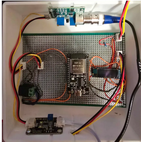
FIGURE 8.1. Vue intérieure du boîtier — prototype sur veroboard
