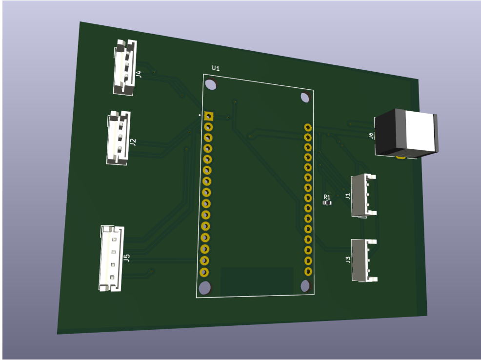
FIGURE 4.3. Rendu 3D de la carte aqua-ai-monitor (KiCad 7)
