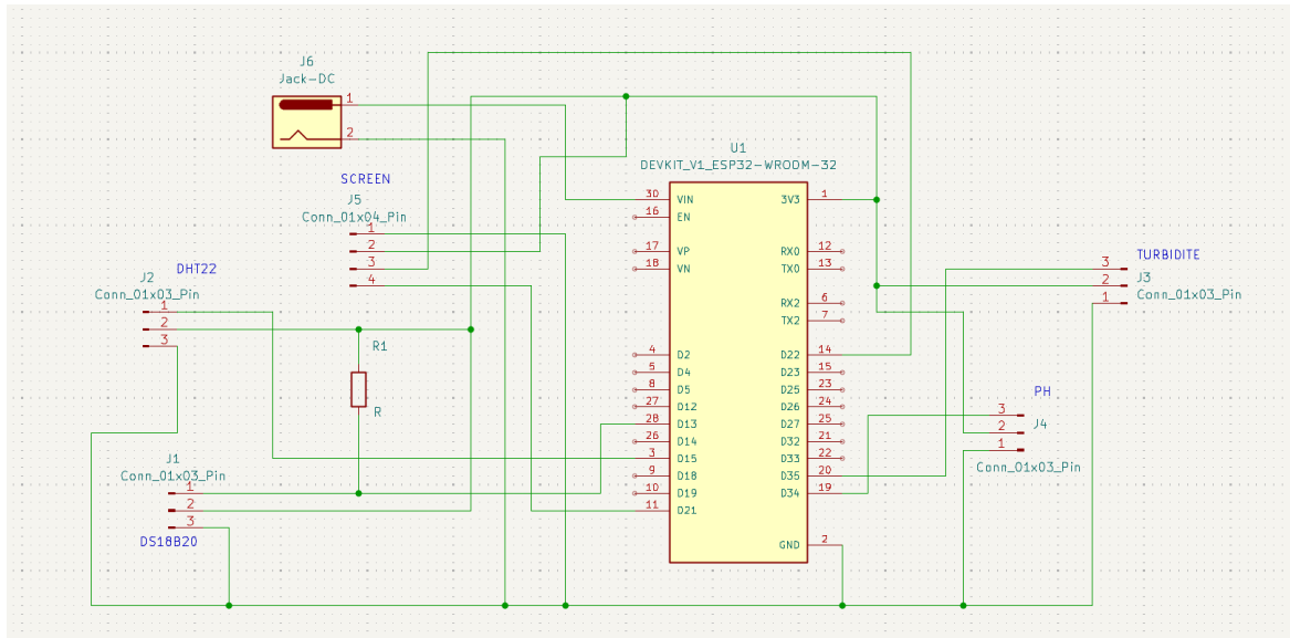
FIGURE 4.1. Schématique électronique de la carte aqua-ai-monitor (KiCad 7)
