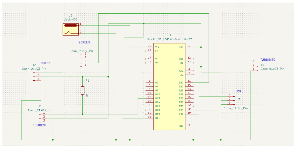
FIGURE 4.1. Schématique électronique de la carte aqua-ai-monitor (KiCad 7)
