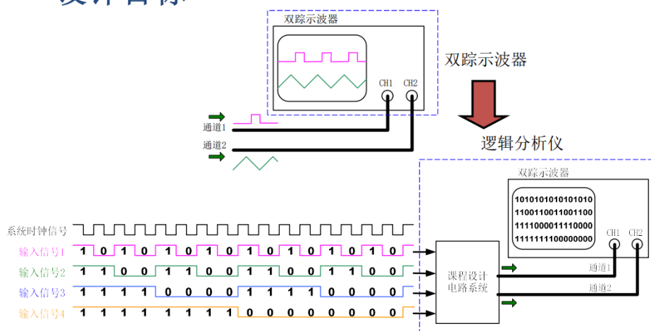
改通用示波器为简易逻辑分析仪
