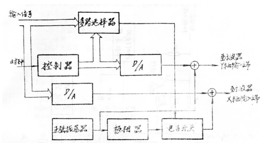
示波器显示逻辑字符功能扩展框图
