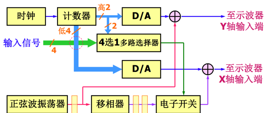
示波器显示逻辑字符功能扩展框图
